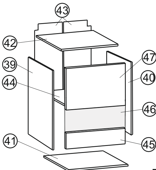
Góra 60/72 / Top 60/72
