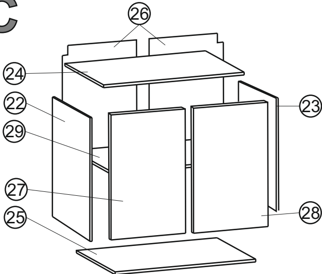
Góra 80/72 / Top 80/72
