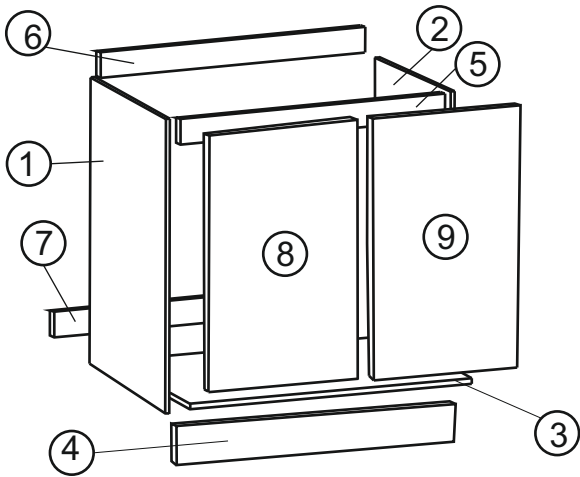
Dół 80 Zlew / Bottom 80 Sink
