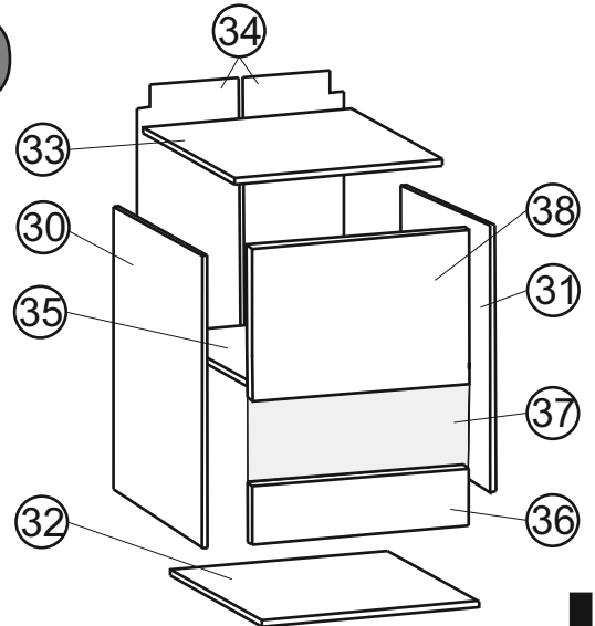
Góra 60/72 / Top 60/72
