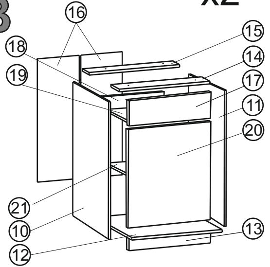
Dół 60 z 1 Szufladą / Bottom 60 with 1 drawer
